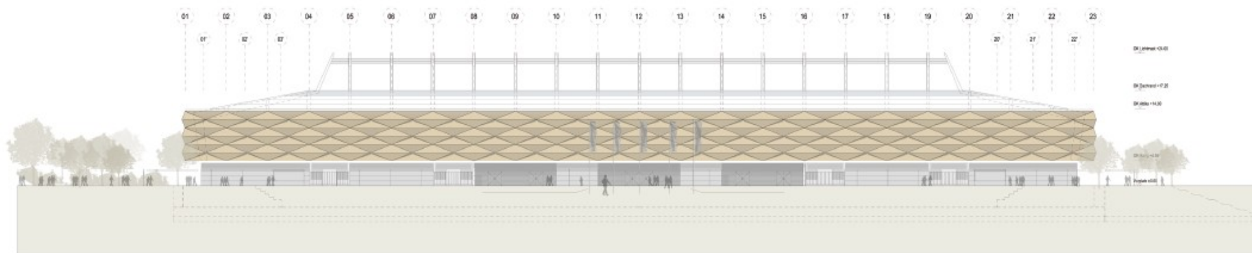
Ansicht Süd | Haupteingang
