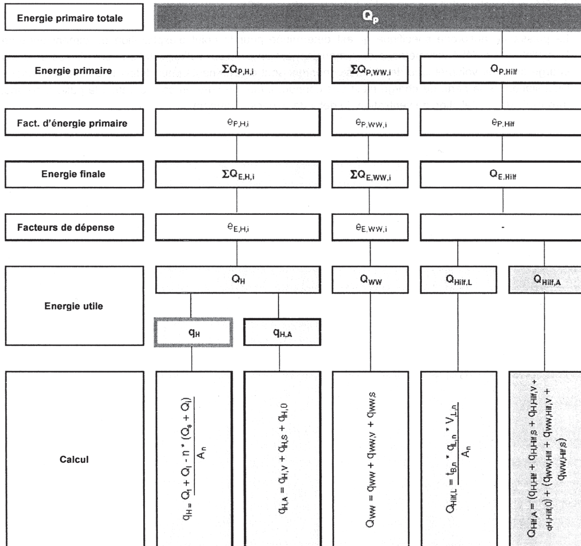
Illustration 1 – Schéma du bilan énergétique des bâtiments d'habitation
