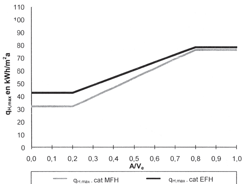
Illustration 2b – Exigences relatives à la valeur spécifique du besoin en chaleur de chauffage pour les bâtiments d'habitation dont l'autorisation de bâtir est demandée à partir du 1er juillet 2012 et jusqu'au 31 décembre 2014
