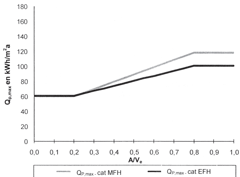
Illustration 3b – Exigences relatives à la valeur spécifique du besoin en énergie primaire pour les bâtiments d'habitation dont l'autorisation de bâtir est demandée à partir du 1er juillet 2012 et jusqu'au 31 décembre 2014
