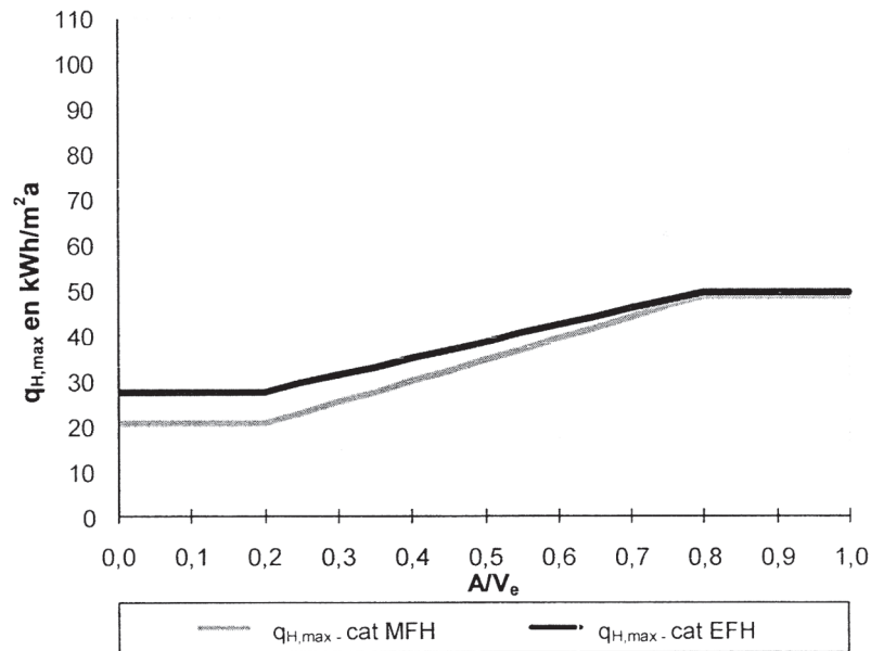
Illustration 2c – Exigences relatives à la valeur spécifique du besoin en chaleur de chauffage pour les bâtiments d'habitation dont l'autorisation de bâtir est demandée à partir du 1er janvier 2015 et jusqu'au 31 décembre 2016
