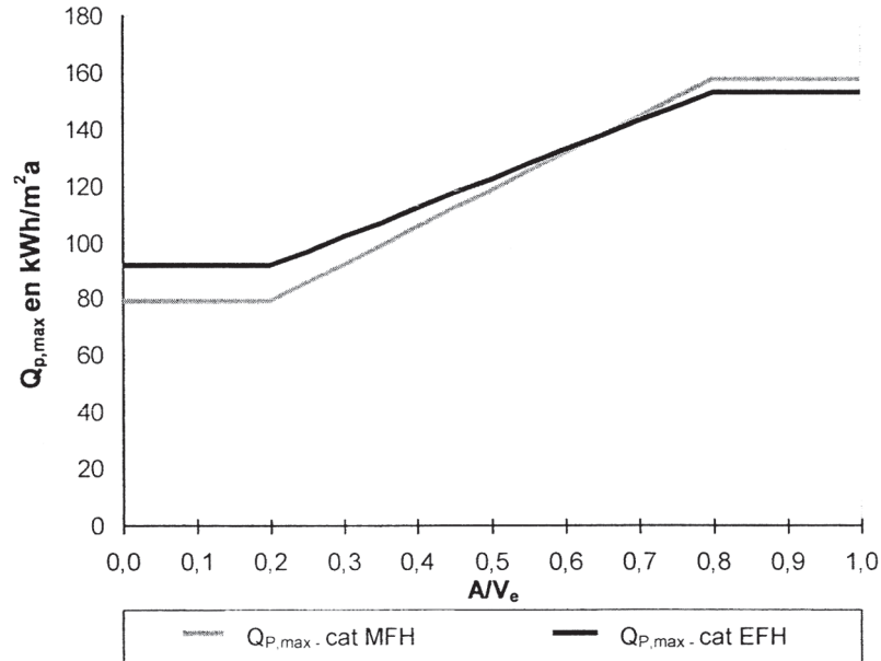
Illustration 3a – Exigences relatives à la valeur spécifique du besoin en énergie primaire pour les bâtiments d'habitation dont l'autorisation de bâtir est demandée jusqu'au 30 juin 2012
