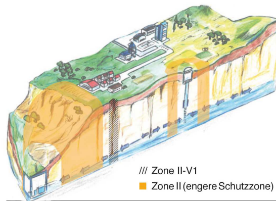
EINTEILUNG DER ZONE II UND II-V1
