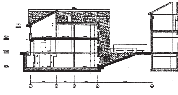
COUPE B-B
