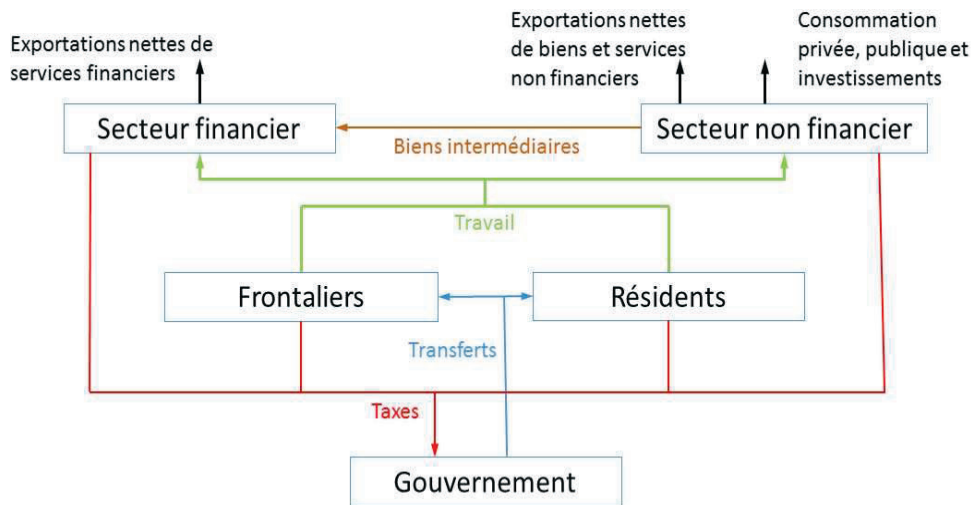
Graphique 37 : Représentation simplifiée du modèle LOLA3
