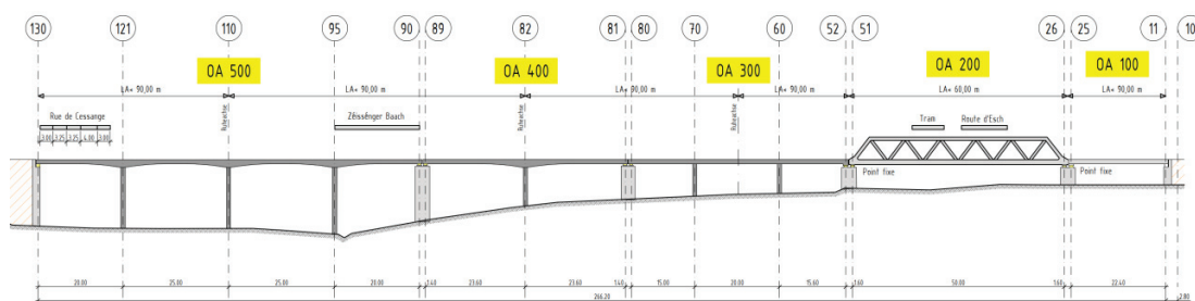
Figure 10: Coupe longitudinale des différents ouvrages de franchissement
