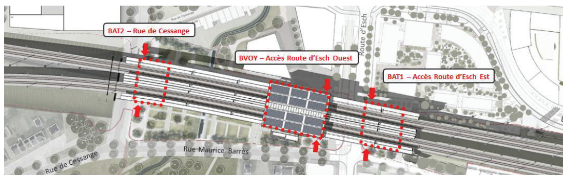
Figure 6: Implantation des quais et des bâtiments d'accès
