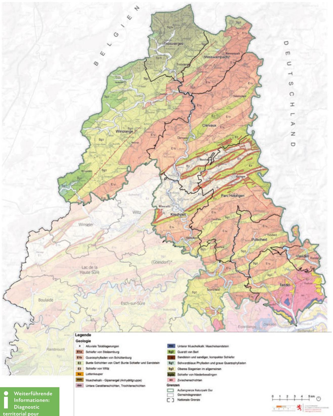
Abb. 8 - Geologische Karte des Naturpark Our (Quelle: Open Data WMS and WMTS / Administration du cadastre et de la topographie du Grand-Duché du Luxembourg, Darstellung : DATer, pact s.à.r.l.)
