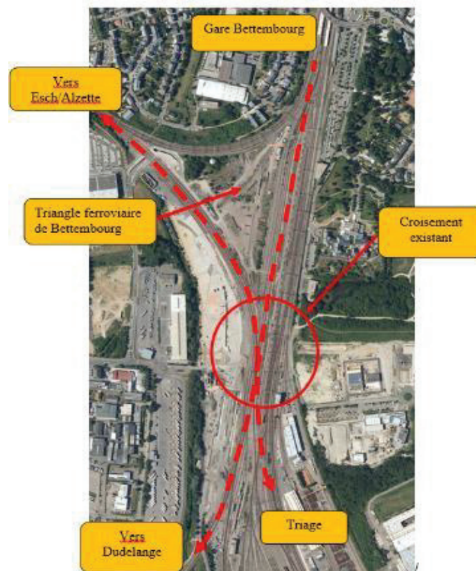
Figure – Implantation du Saut de Mouton
