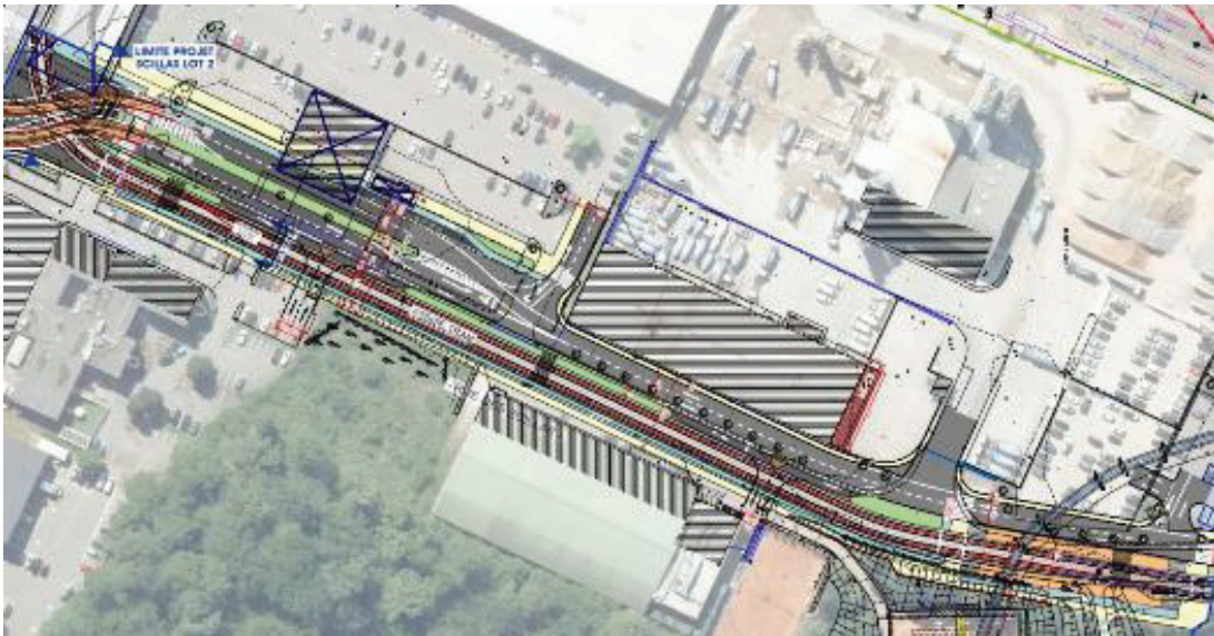
Figure 5 : Plan d'aménagement au stade d'Exécution
