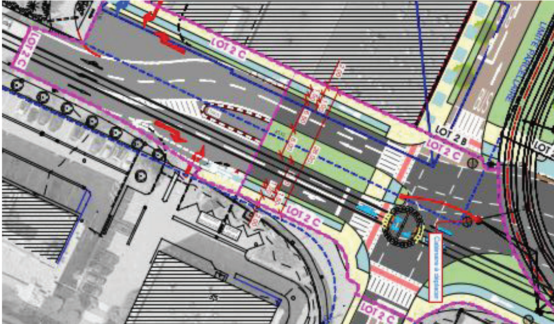
Figure 7 : Plan de situation au stade de la soumission de la rue des Scillas entre la rue des Bruyères et le boulevard Raiffeisen.
